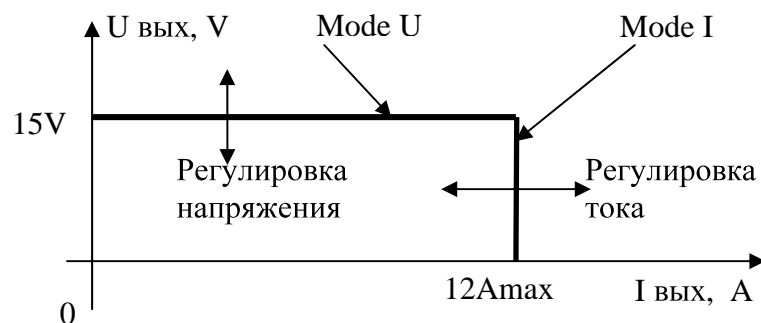
Рис. 2. Вольт-амперная характеристика источника питания
